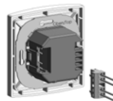
steckbare Schraubklemmen
